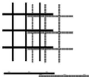
Traslapes en zonas en que el acero trabaja a menos de la mitad del esfuerzo permisible.
